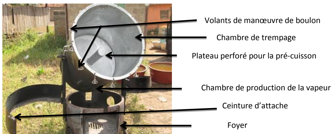
Figure 1 : Kit d'étuvage de 180kg (KIT 180- riz)
